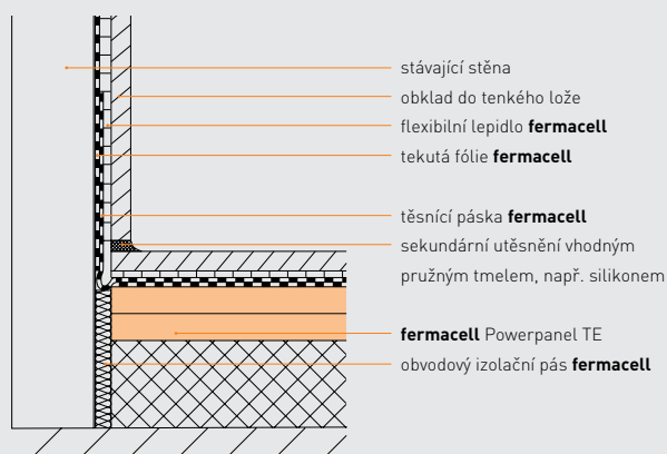
Napojení stěna – potěr v oblasti namáhané vodou
