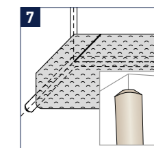
H204 Rohový profil CA12 pro stěnové fabion
